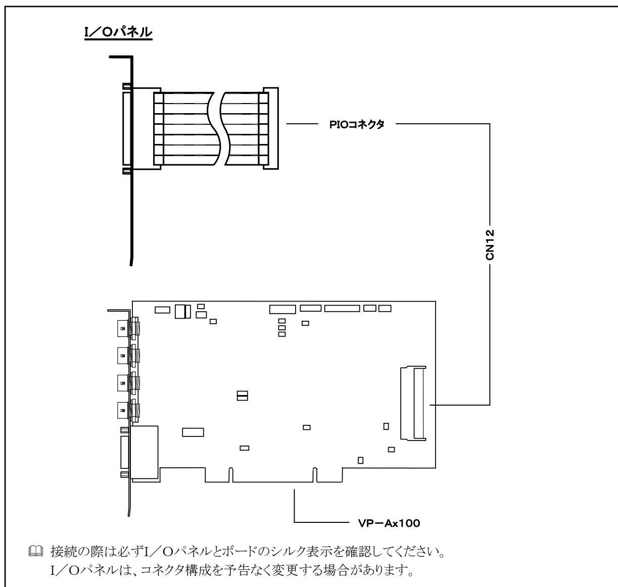
図1-7 I/Oパネルの接続図
