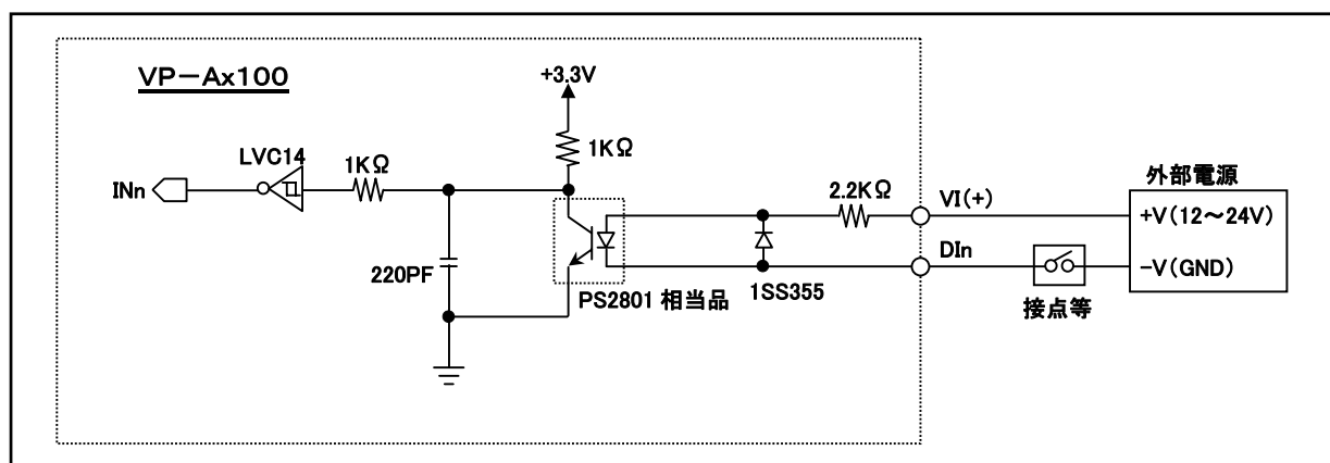
図2-9 入力回路図
