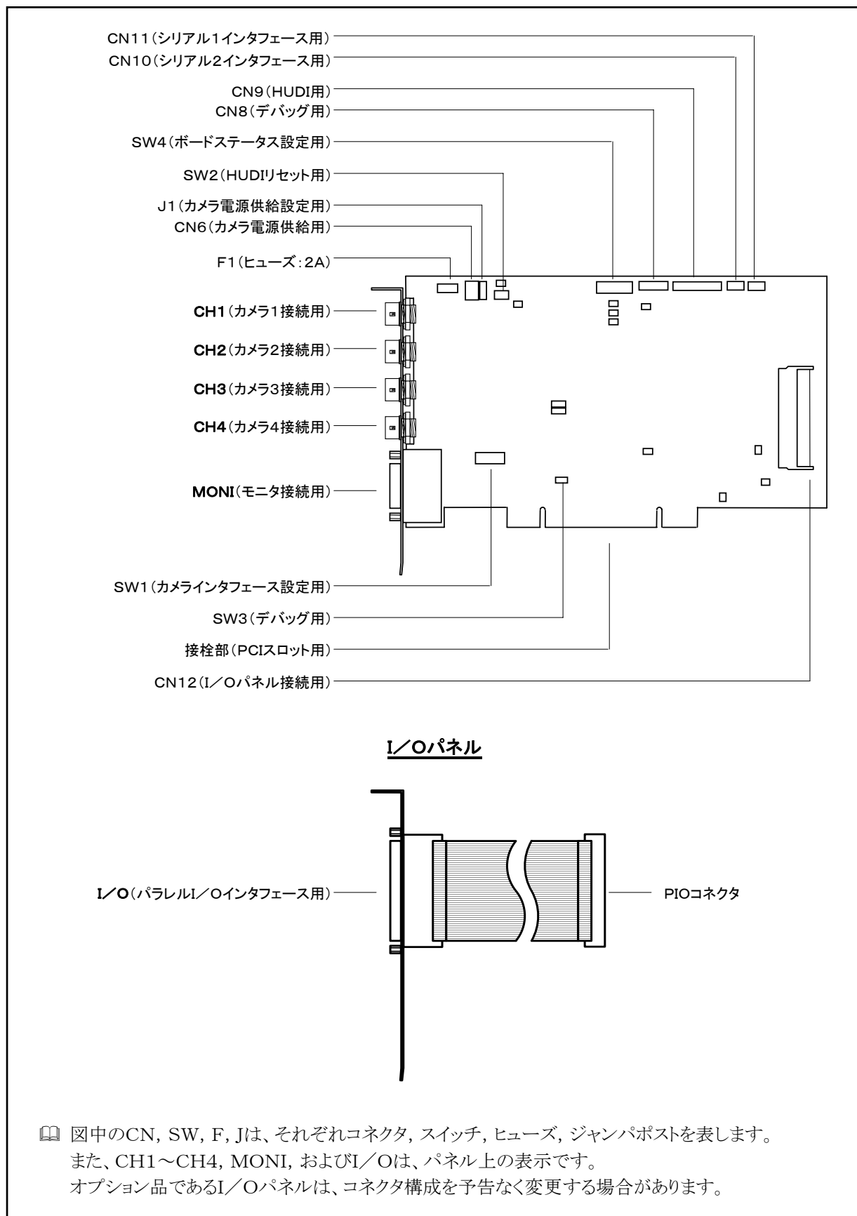
図1-2 各部の名称
