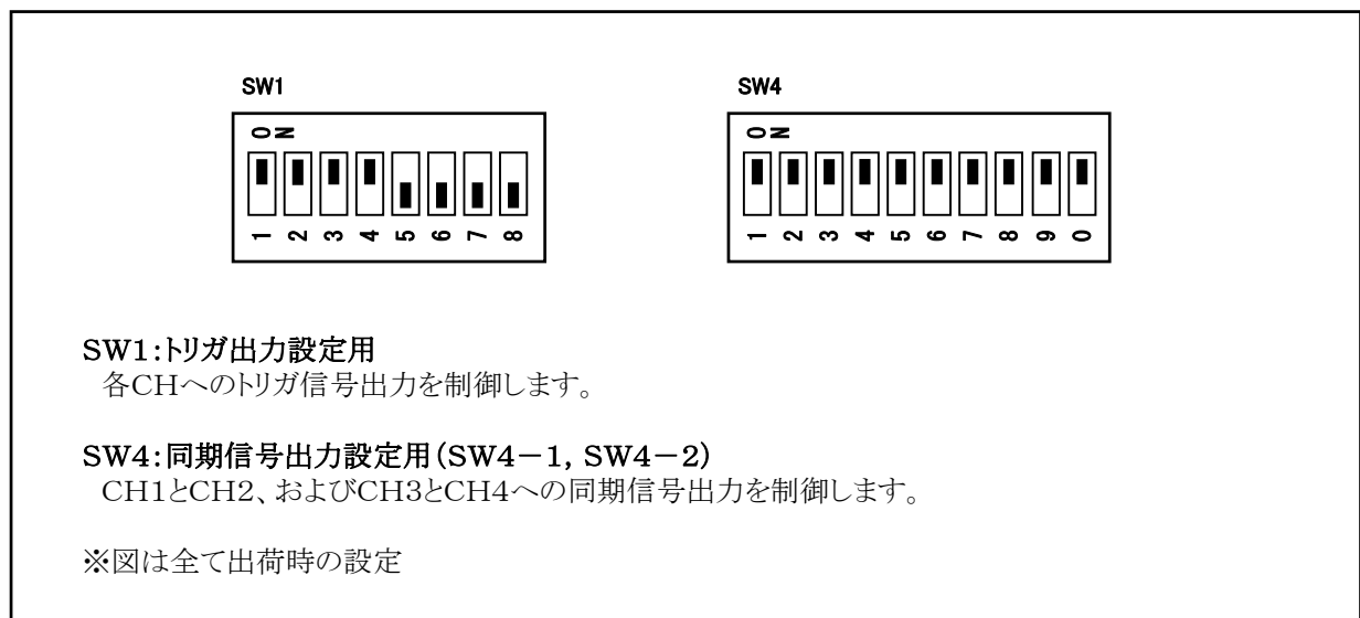
図1-5 カメラインタフェース設定の概要
