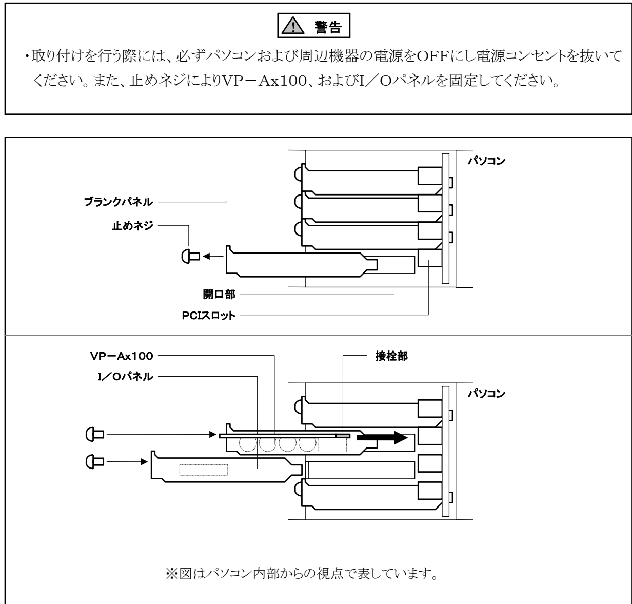
図1-8 VP-Ax100の取り付け図
