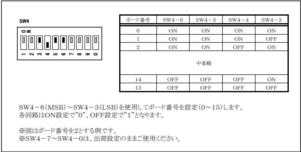
図1-6 ボードステータス設定 (SW4) の詳細
