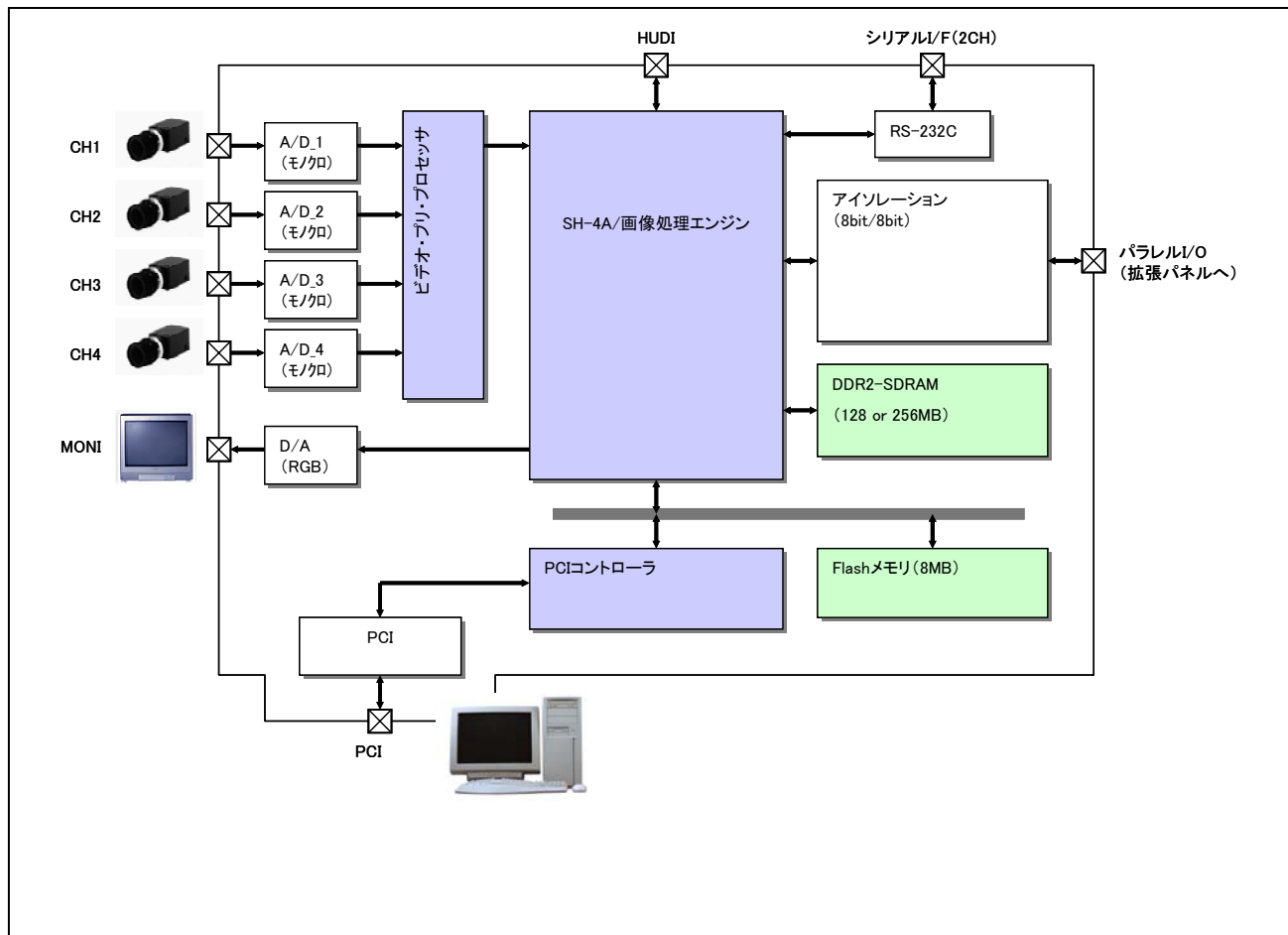
図2-1 ブロック図
