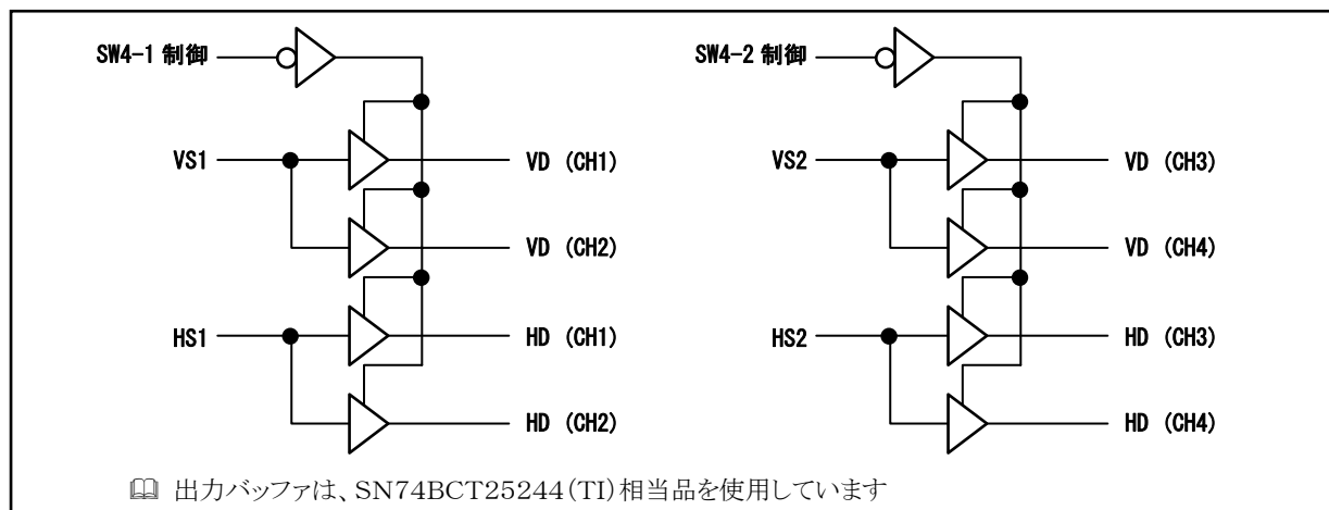
図2-4 カメラ外部同期信号出力回路
