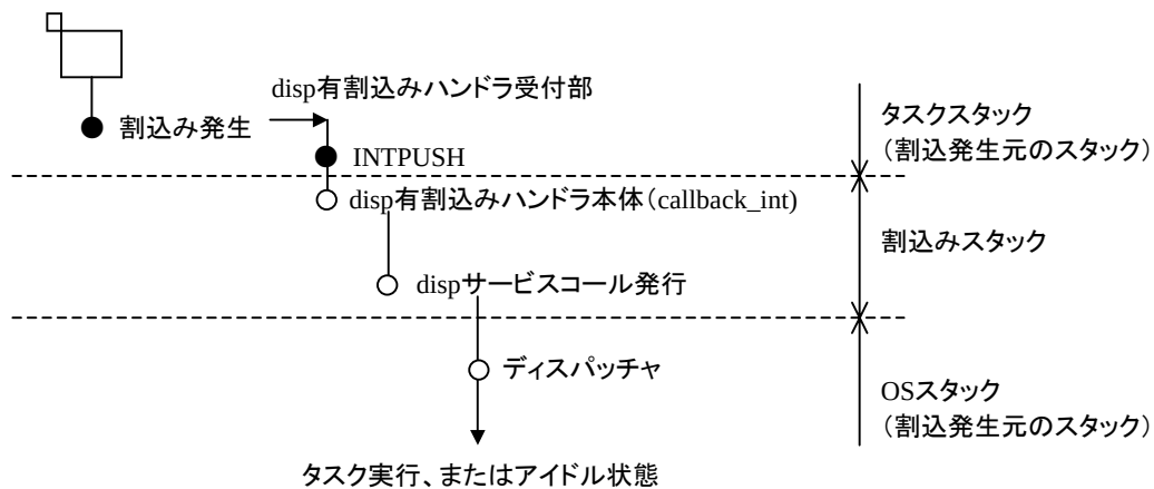
図6-6 disp有割込みハンドラのスタック切り替えタイミング
