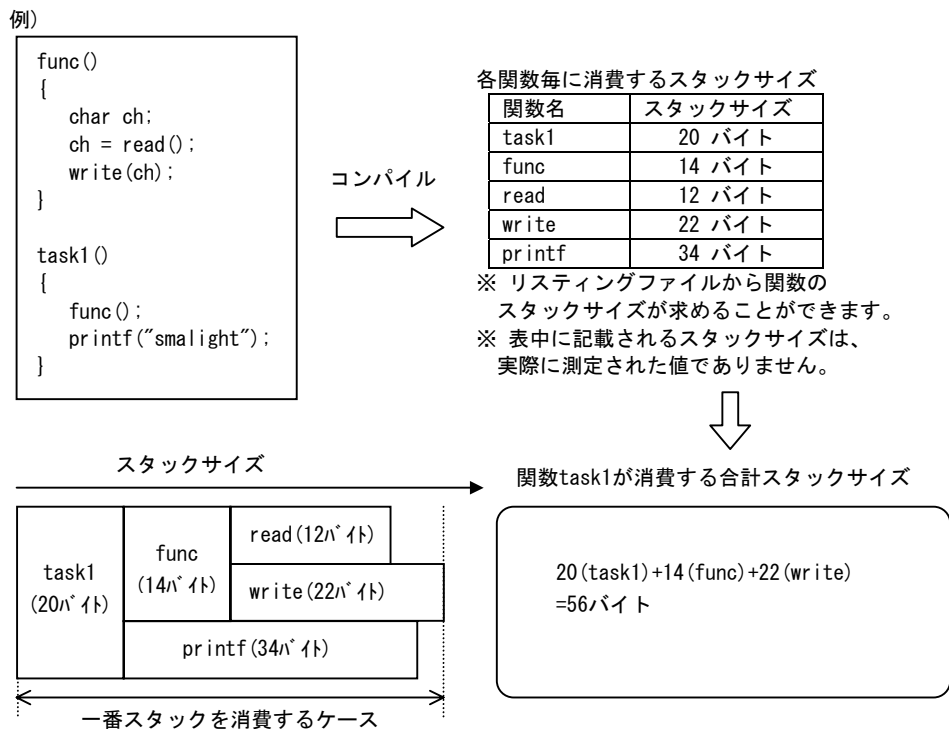
図6-3 関数のスタック計算方法
