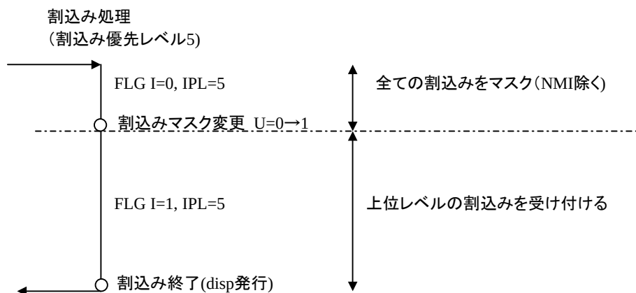
図3-19 多重割込み実現方式の例
