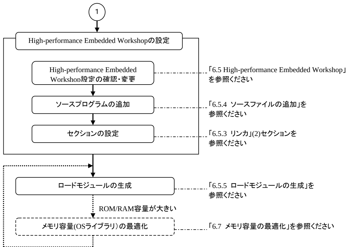
図6-2 構築手順②
