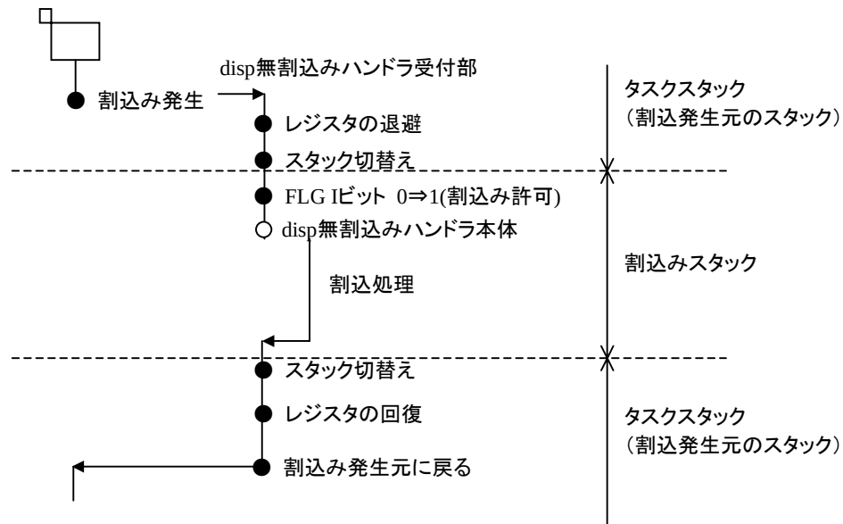
図6-5 disp無割込みハンドラのスタック切り替えタイミング
