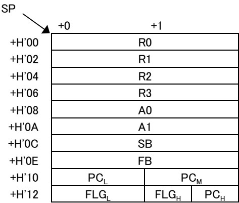
図C-1 M16C/2x,3x,6xグループのスタック仕様
