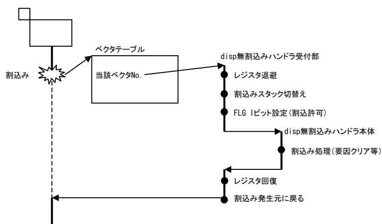
図3-14 disp無割込みハンドラの基本動作
