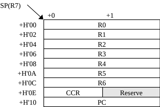
図C-1 H8/300Lのスタック仕様
