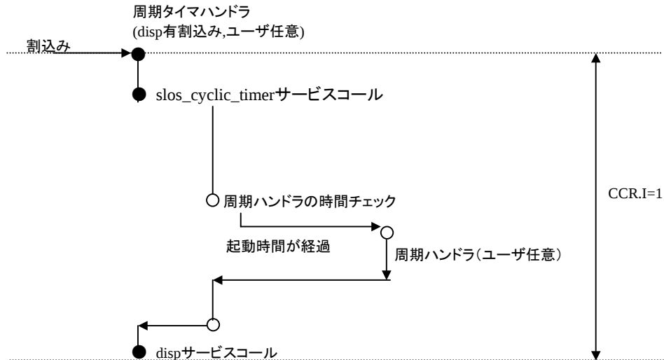
図3-13 周期ハンドラの呼び出し
