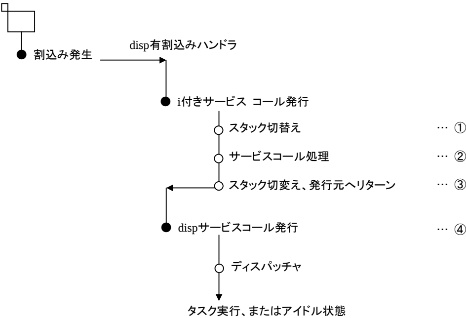
図4-2 i 付きサービスコールの基本動作
