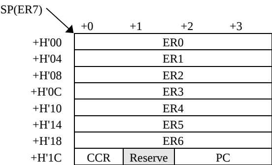
図C-1 H8/300H Normalモード時のスタック仕様
