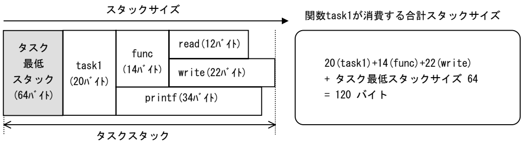
図6-4 タスクのスタック計算方法
