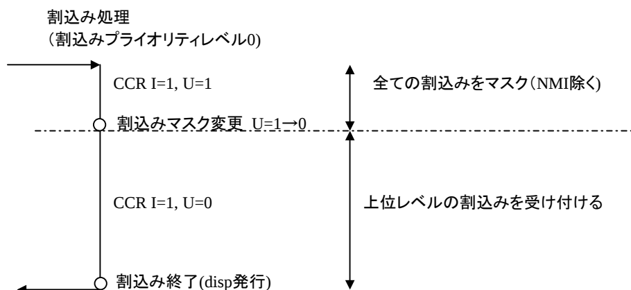
図3-19 多重割込み実現方式
