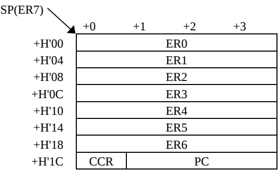
図C-2 H8/300H Advancedモード時のスタック仕様
