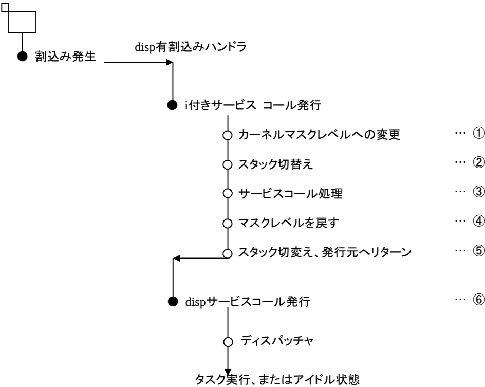
図4-2 i 付きサービスコールの基本動作
