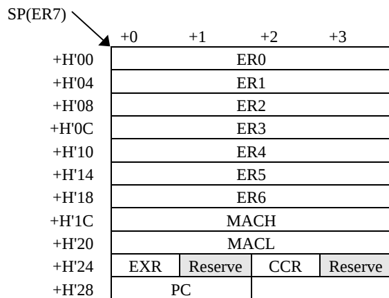
図C-2 H8S/2600 Normalモード(割込制御モード2、3時)のスタック仕様
