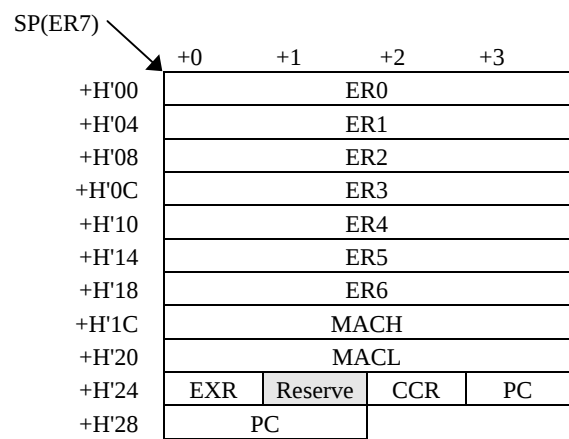
図C-4 H8S/2600 Advancedモード(割込制御モード2、3時)のスタック仕様
