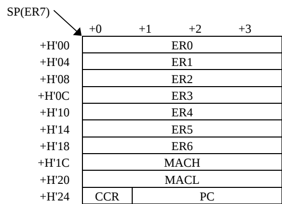
図C-3 H8S/2600 Advancedモード(割込制御モード0、1時)のスタック仕様
