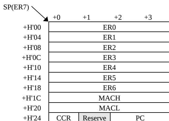
図C-1 H8S/2600 Normalモード(割込制御モード0、1時)のスタック仕様
