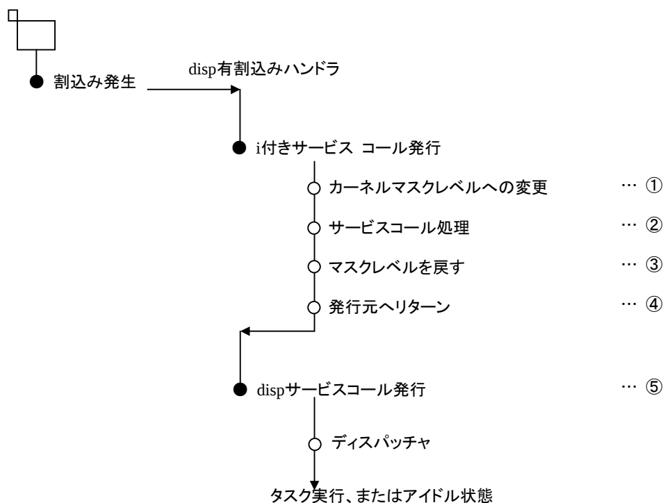
図4-3 i付きサービスコールの基本動作(割込みモード2,3)
