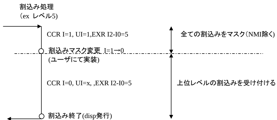
図3-21 多重割込み実現方式①(割込み制御モード3)
