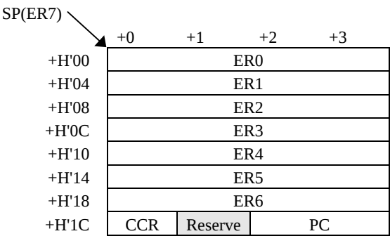
図C-1 H8S/2000 Normalモード(割込制御モード0、1時)のスタック仕様
