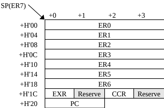
図C-2 H8S/2000 Normalモード(割込制御モード2、3時)のスタック仕様
