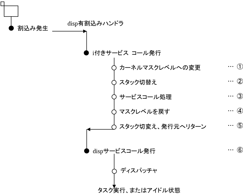
図4-2 i 付きサービスコールの基本動作(割込みモード0,1)
