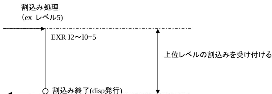
図3-20 多重割込み実現方式(割込み制御モード2)
