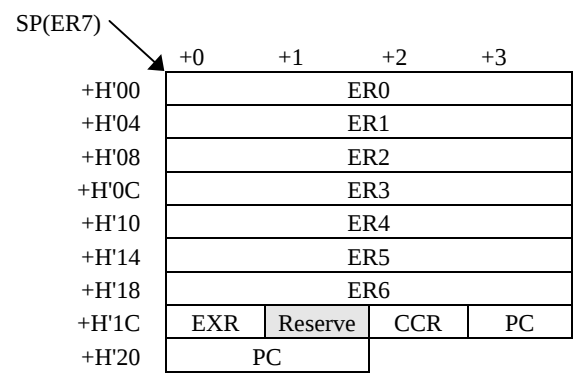
図C-4 H8S/2000 Advancedモード(割込制御モード2、3時)のスタック仕様
