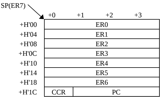
図C-3 H8S/2000 Advancedモード(割込制御モード0、1時)のスタック仕様
