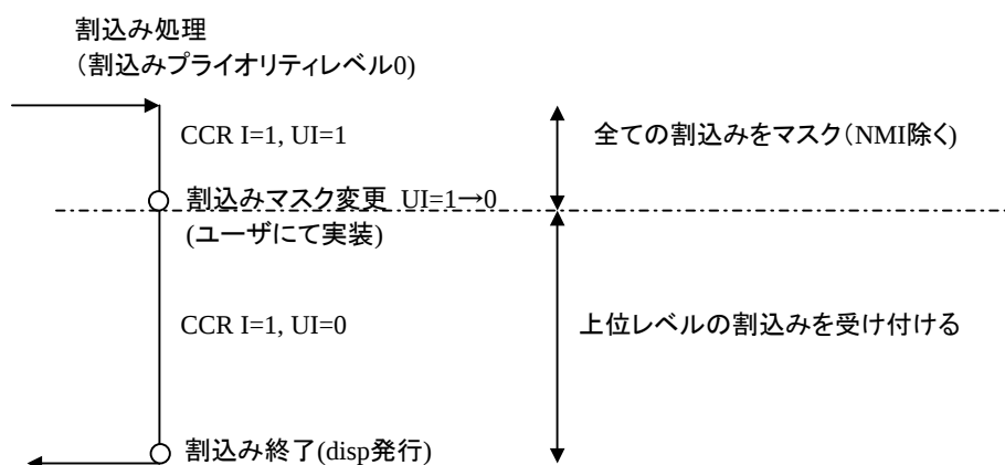
図3-19 多重割込み実現方式(割込み制御モード1)
