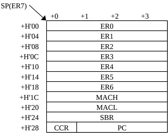
図C-1 H8SX Advancedモード(割込制御モード0時)のスタック仕様
