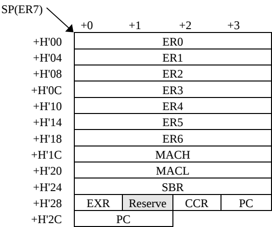
図C-2 H8SX Advancedモード(割込制御モード2時)のスタック仕様
